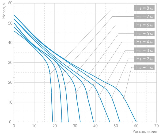
«ДЖАМБО ПРО» 70/50 П (Н)
