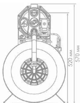
«ДЖАМБО ПРО» 70/50 Н-50 (арт. 3124)
