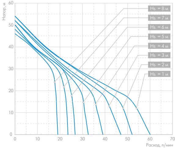
«ДЖАМБО» 70/50 П (Н)
