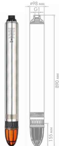
«ВОДОМЕТ» 55/90 (арт. 5590)
