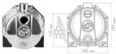
«ДЖАМБО ПРО» 70/50 Н (арт. 3104)
