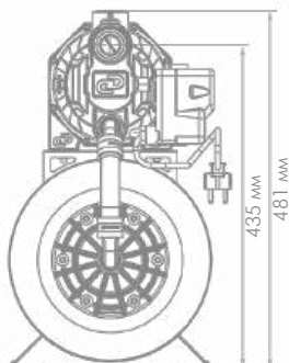
«ДЖАМБО ПРО» 60/35 П-24 (арт. 3111)
