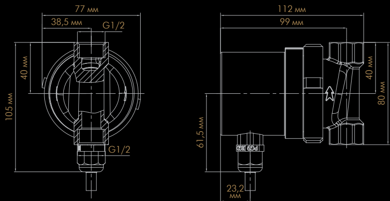
Пример обозначения: «ЦИРКУЛЬ» 15*/15** PREMIUM * условное проходное сечение насоса, мм; ** максимальный напор (с учетом округления) водяного столба, дм.
