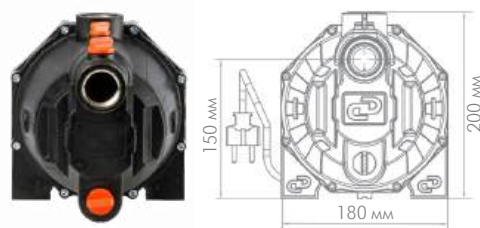
«ДЖАМБО ПРО» 70/50 П (арт. 3102)
