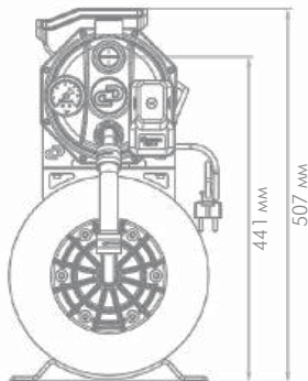
«ДЖАМБО» 70/50 Н-24 (арт. 3712)
