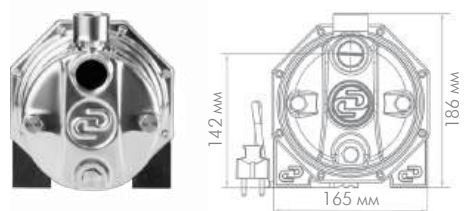
«ДЖАМБО ПРО» 60/35 Н (арт. 3103)
