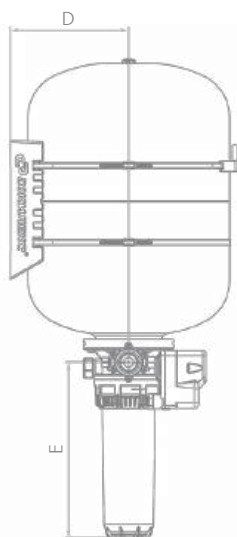
КРАБ 50 (арт. 9030)
