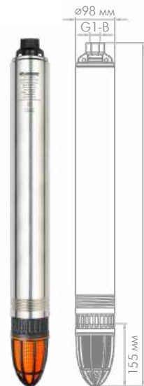
«ВОДОМЕТ» 75/75 (арт. 7575)
