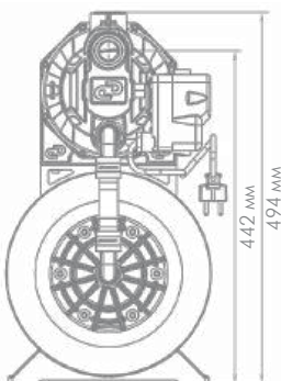
«ДЖАМБО ПРО» 70/50 П-24 (арт. 3112)
