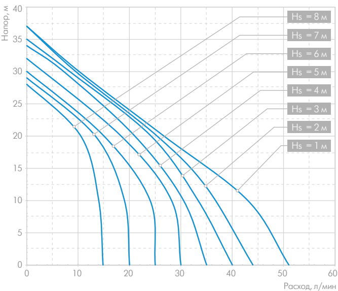
«ДЖАМБО ПРО» 60/35 П (Н)
