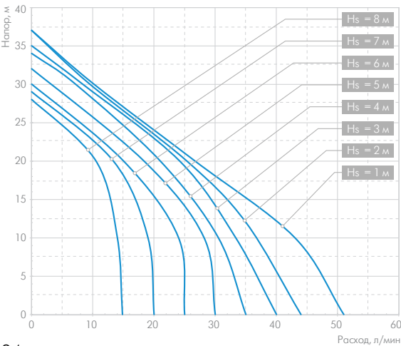
«ДЖАМБО» 60/35 П (Н)
