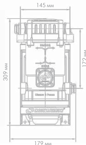
«КОМФОРТ ПРО» 25/16 (арт. 4003)
