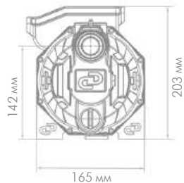
«ДЖАМБО» 60/35 Ч (арт. 3005)
