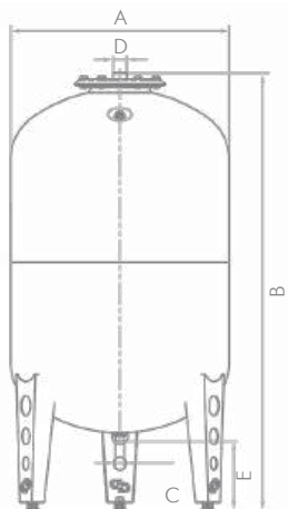
Расширительный бак B 50 (арт. 7750)
