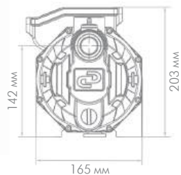
«ДЖАМБО» 60/35 П (арт. 3004)
