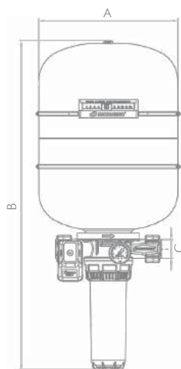
КРАБ 24 (арт. 9029)
