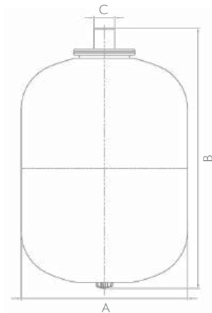
Расширительный бак В 14 (арт. 7814)
