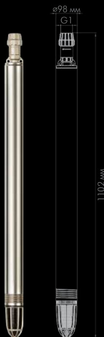
«ВОДОМЕТ 3Д» 55/70 PREMIUM (арт. 6870)
