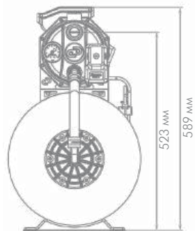
«ДЖАМБО» 70/50 Н-50 (арт. 3722)
