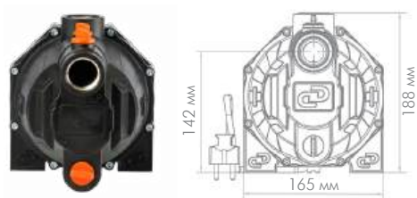
«ДЖАМБО ПРО» 60/35 П (арт. 3101)
